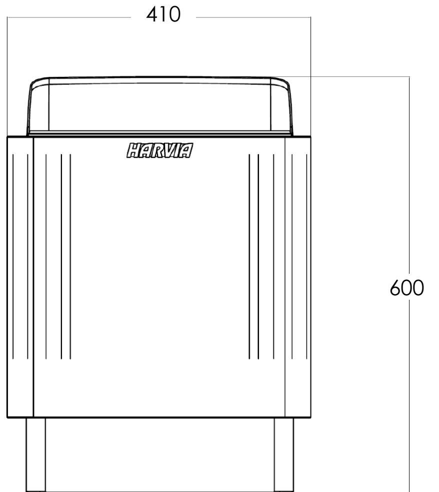
正面図
