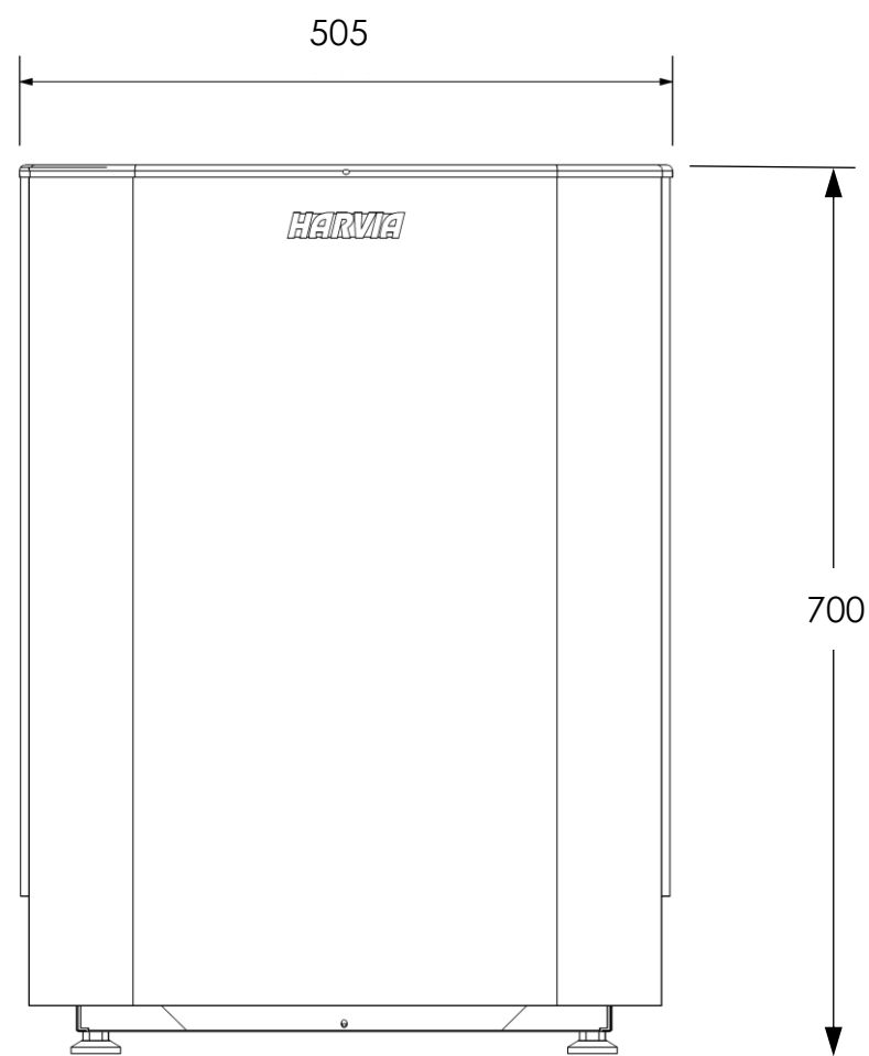
正面図
