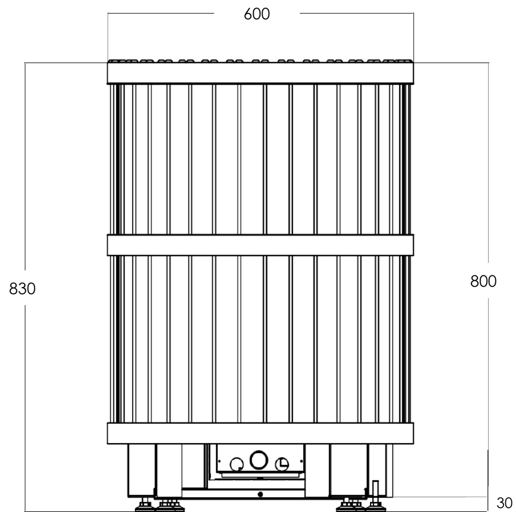
正面図
