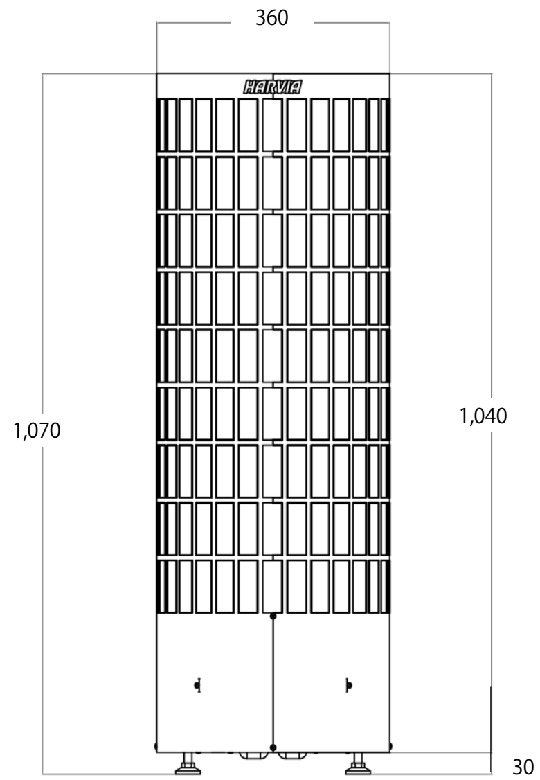
正面図
