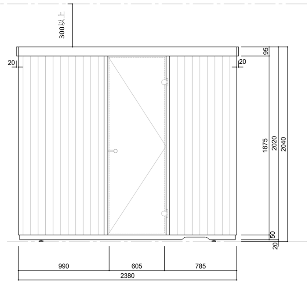
正面図
