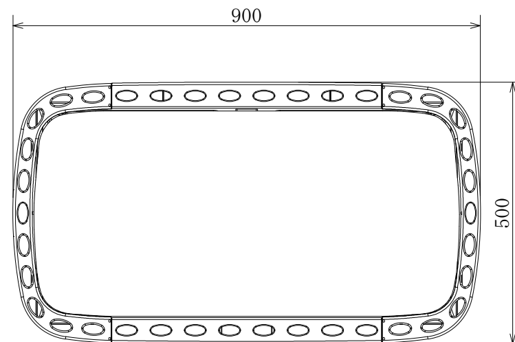
上面図
