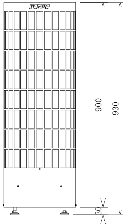
正面図
