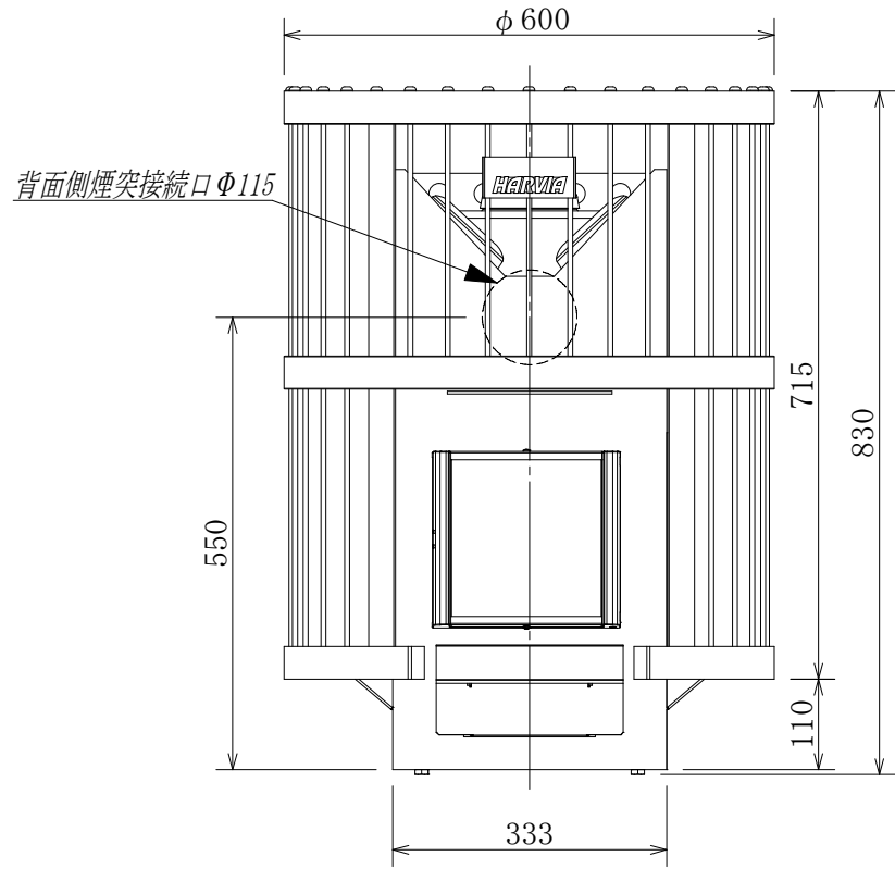
正面図
