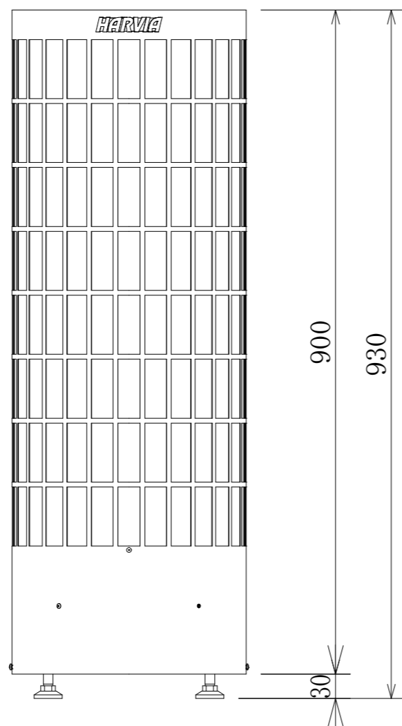
正面図
